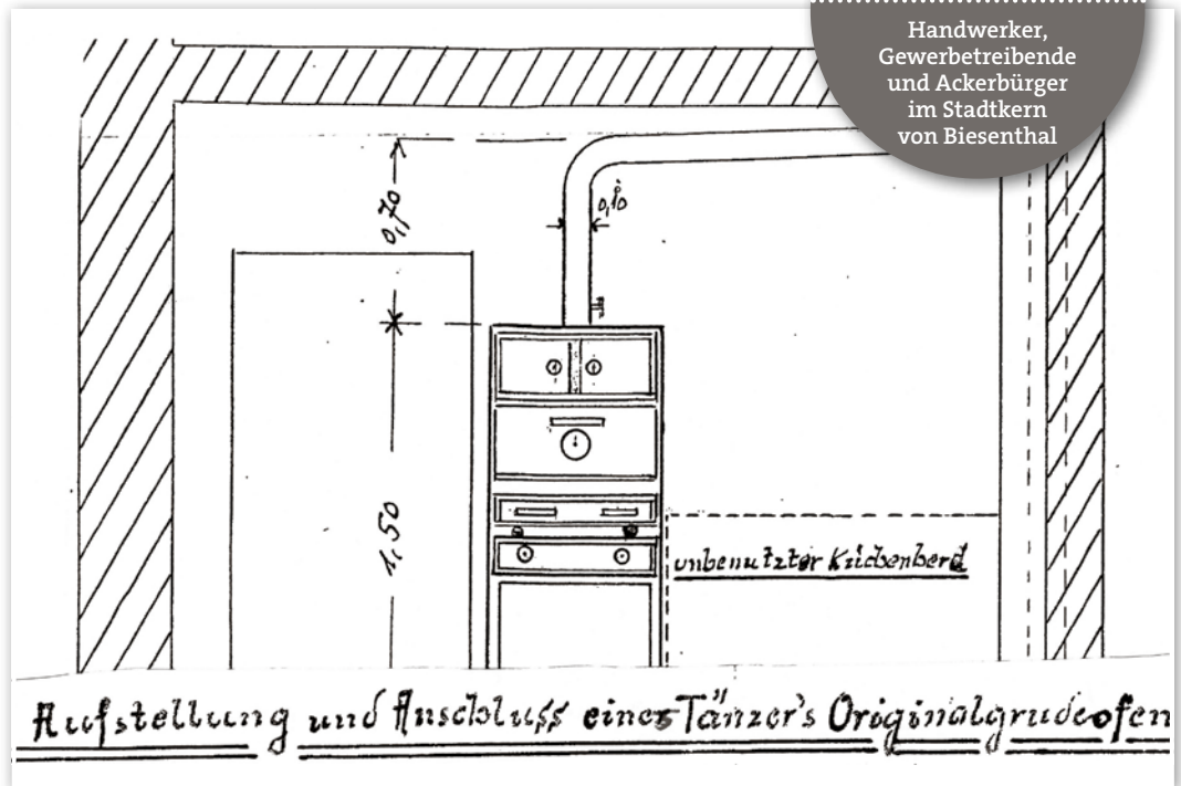
Eine Zeichnung vom „Grudeofen“, den Herr Richard Vogel 1938 in seiner Küche einbauen ließ
