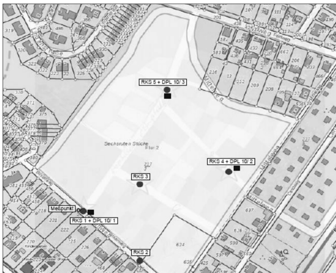
Abbildung 3: Markierung der Bohrpunkte, Geotechnischer Bericht, 2017
