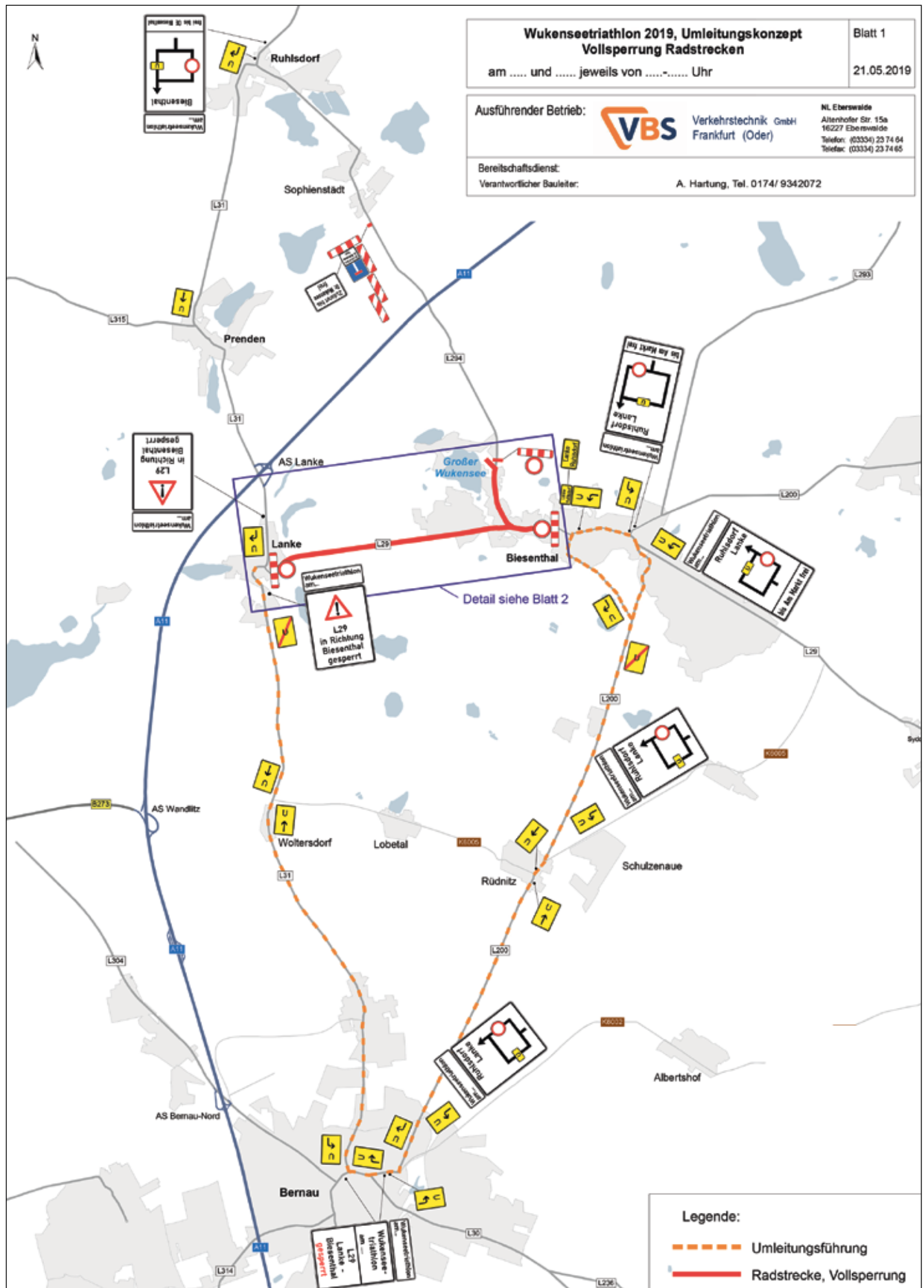
Anlage: Umleitungsplan
