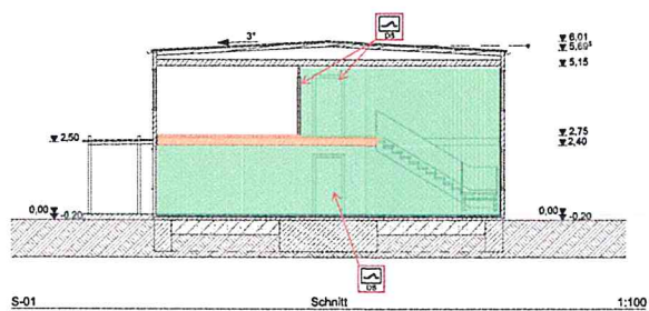
S-01 Schnitt 1:100
