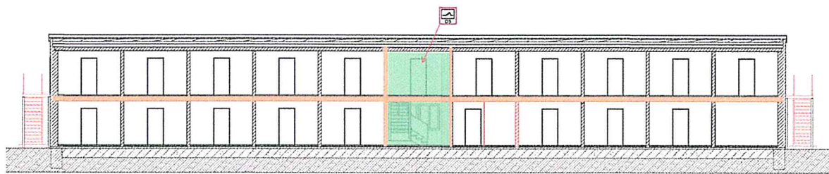
S-02 Schnitt 1:100
